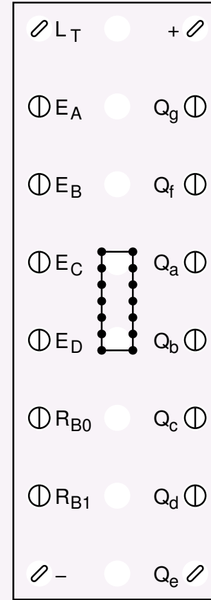
SN 7447 grün green vert
